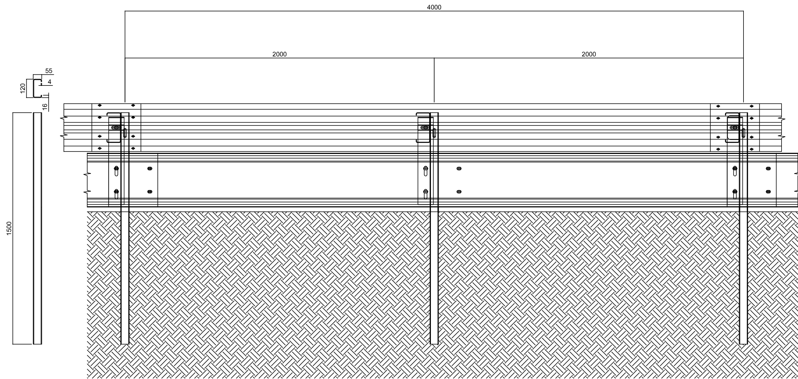
Sezione Orizzontale
